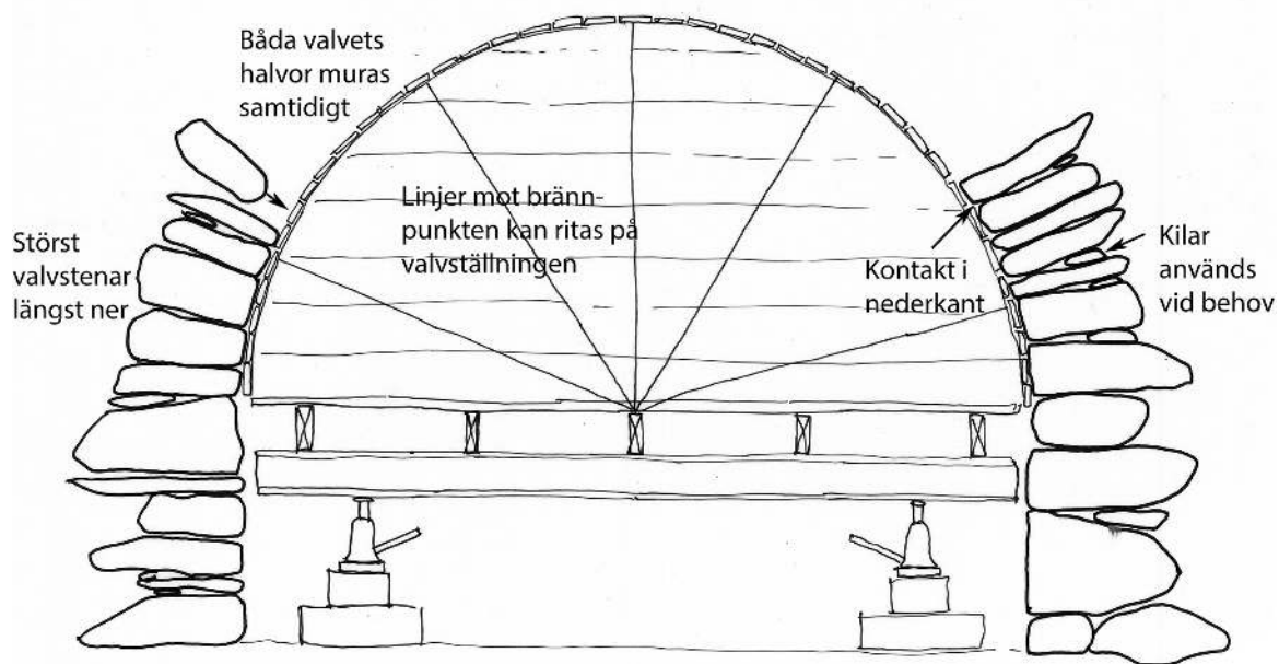
Princip för murning av valv. I den här valvställningen används hydrauliska domkrafter för höjning och sänkning. Förr användes vanligast långa kilar för att sänka ställningen när valvet murats färdigt.
